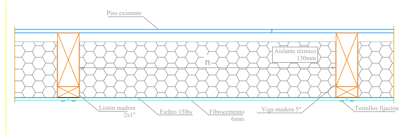
DETALLE SOLUCIÓN CONSTRUCTIVA Escala S/E
