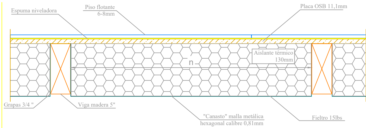
DETALLE SOLUCIÓN CONSTRUCTIVA Escala S/E
