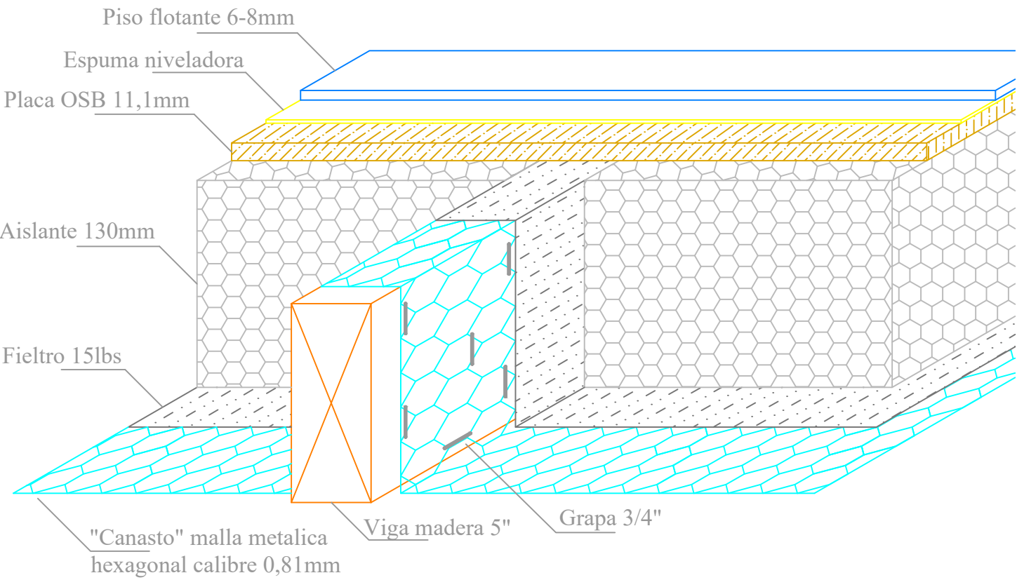
DETALLE ELEMENTOS SOLUCIÓN CONSTRUCTIVA Escala S/E
