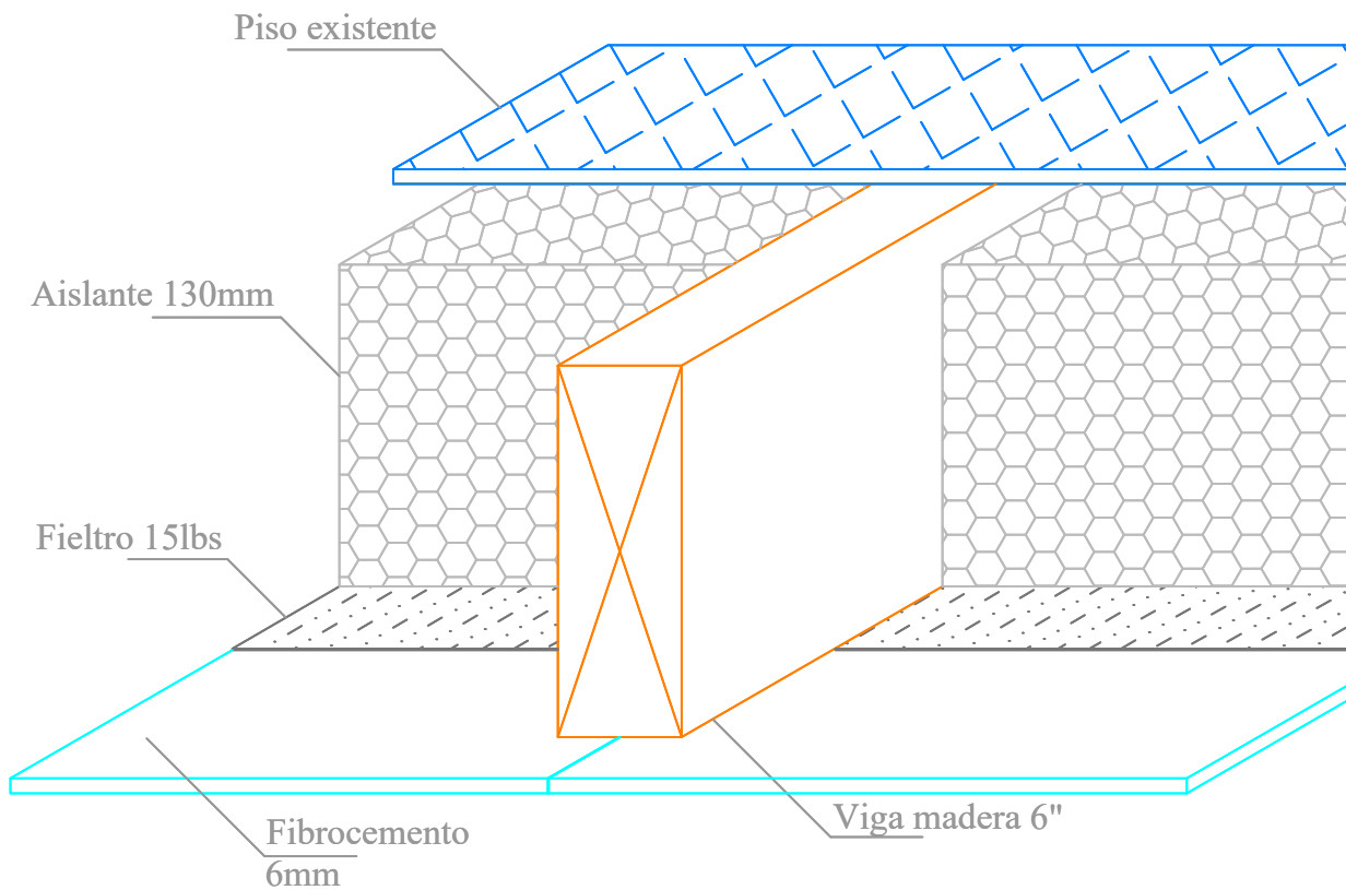
DETALLE ELEMENTOS SOLUCIÓN CONSTRUCTIVA Escala S/E
