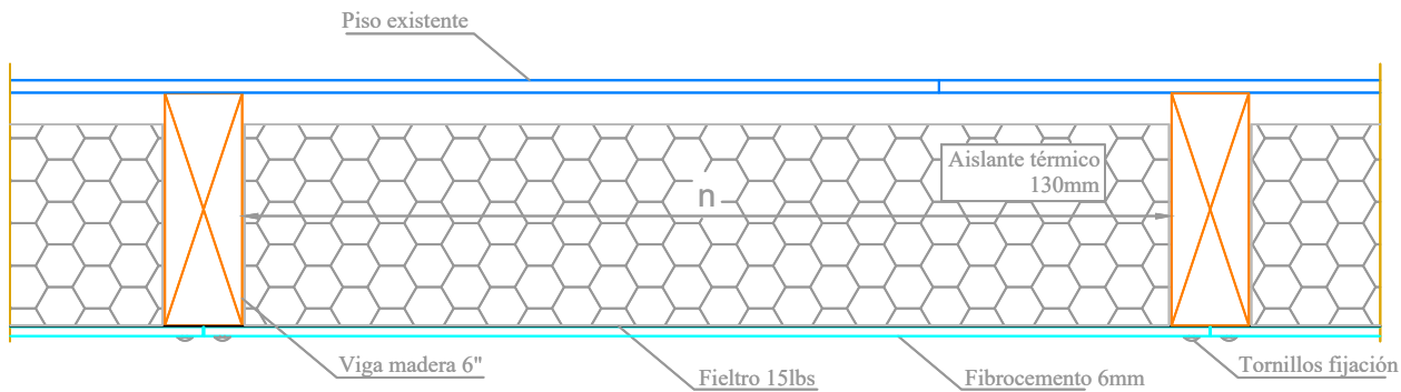
DETALLE SOLUCIÓN CONSTRUCTIVA Escala S/E
